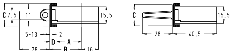
U-vormige voorplaat
